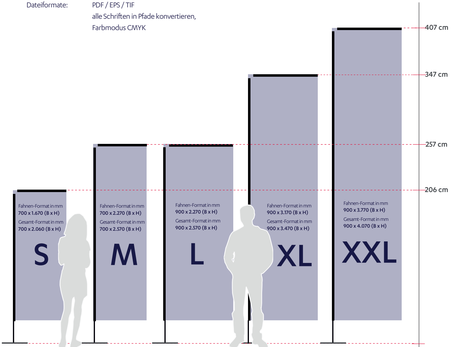
Darstellung im Maßstab 1:30
